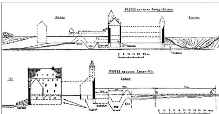
Рис. 6. Замок Георгенбург (рисунок М. Гизе). Расчет уровней поверхности пархама, подвалов и уровня подошвы стен по результатам раскопок 1992-1995 гг. Сплошная линия – уровень современной поверхности; пунктир – предполагаемые уровни пархама, рва и вала.
